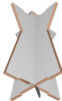
Clamex wird eingeschoben Clamex is inserted Clamex est inséré
